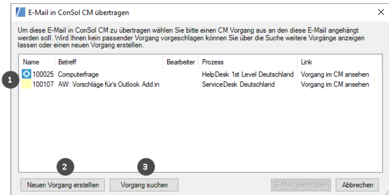
Abbildung 9: Übertragen einer E-Mail
