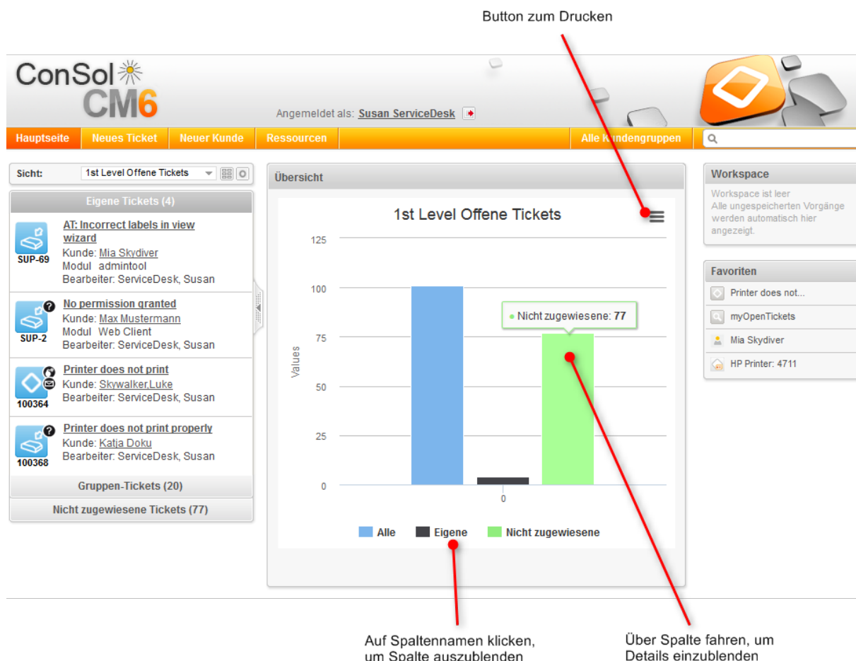
Abbildung 9: Hauptseite mit Dashboard
