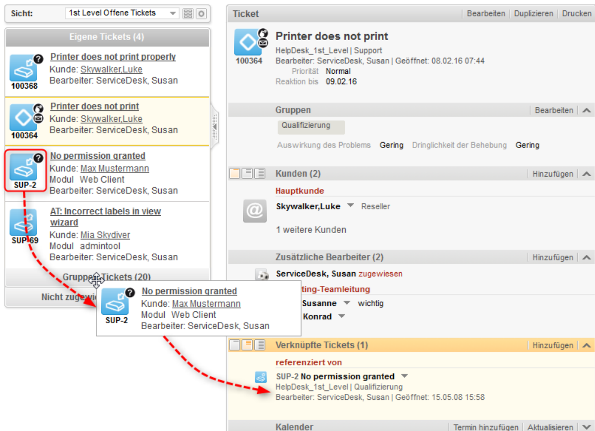
Abbildung 166: Hinzufügen einer Ticketrelation über Drag-and-Drop
