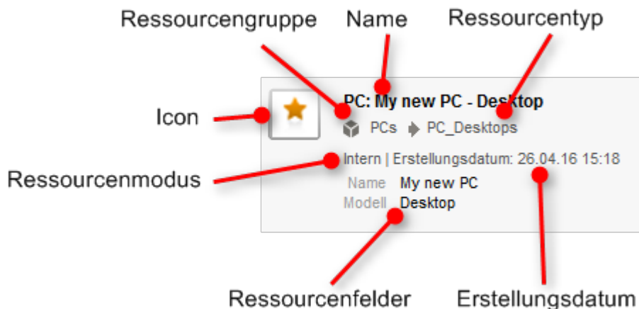
Abbildung 108: Ressourcendaten
