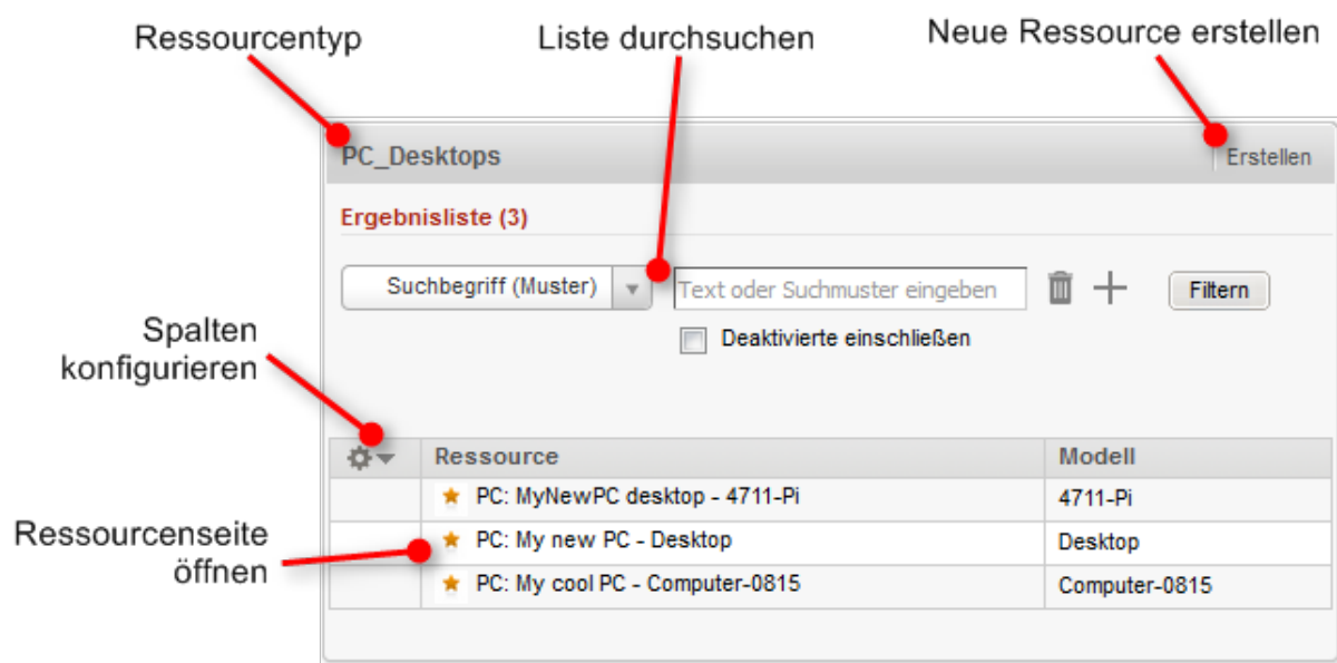
Abbildung 106: Ressourcentyp-Seite
