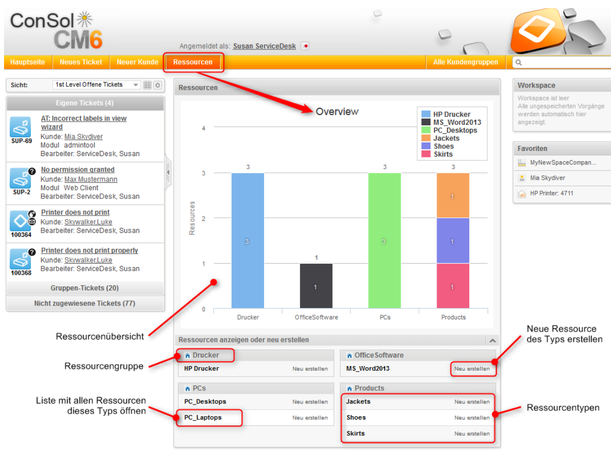
Abbildung 105: Das Ressourcen-Dashboard
