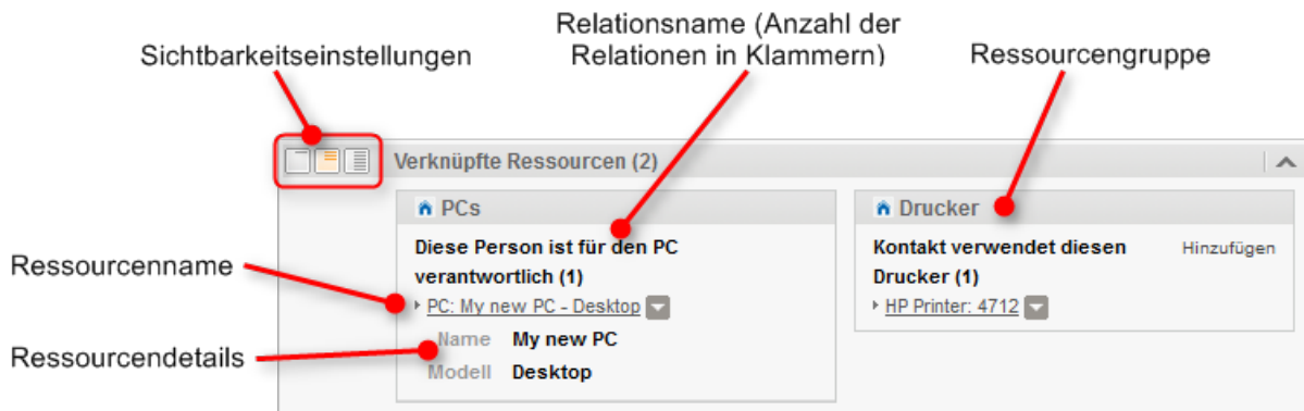
Abbildung 103: Ressourcenrelationen
