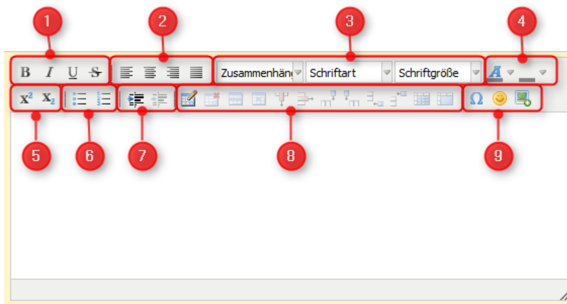
Abbildung 61: Der Rich-Text-Editor
