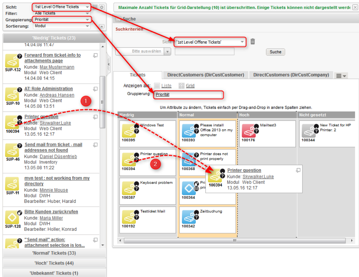
Abbildung 50: Anzeigen der Ticketliste als Grid
