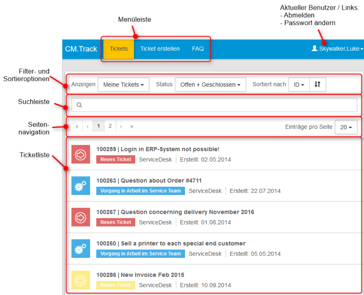
Abbildung 146: Übersichtsseite von CM.Track
