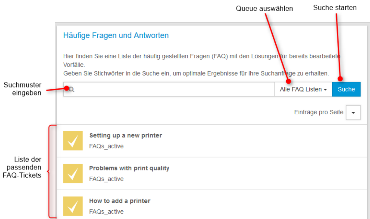
Abbildung 152: Durchsuchen der FAQs
