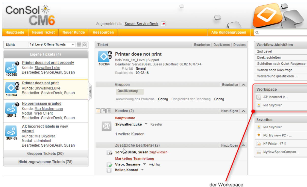
Abbildung 163: Workspace
