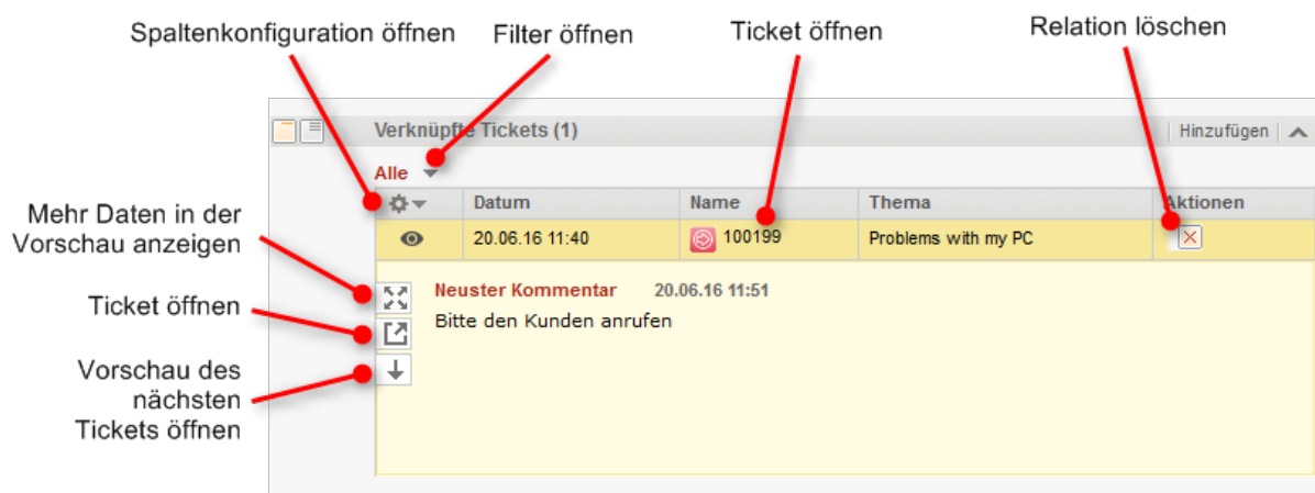
Abbildung 125: Ticketrelationen
