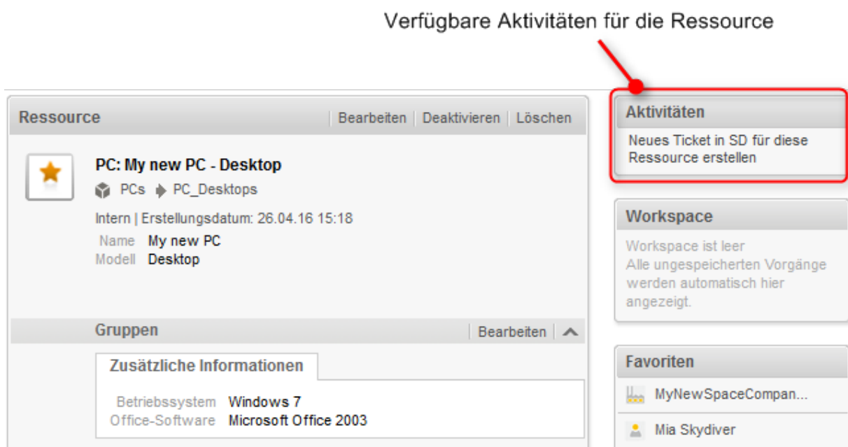
Abbildung 117: Ressourcenaktivitäten
